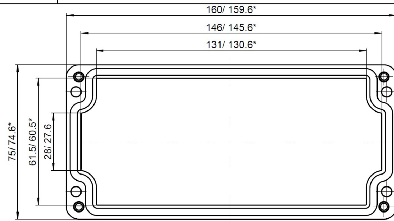
Deckel / Lid
